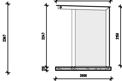
Dwarsdoorsnede
